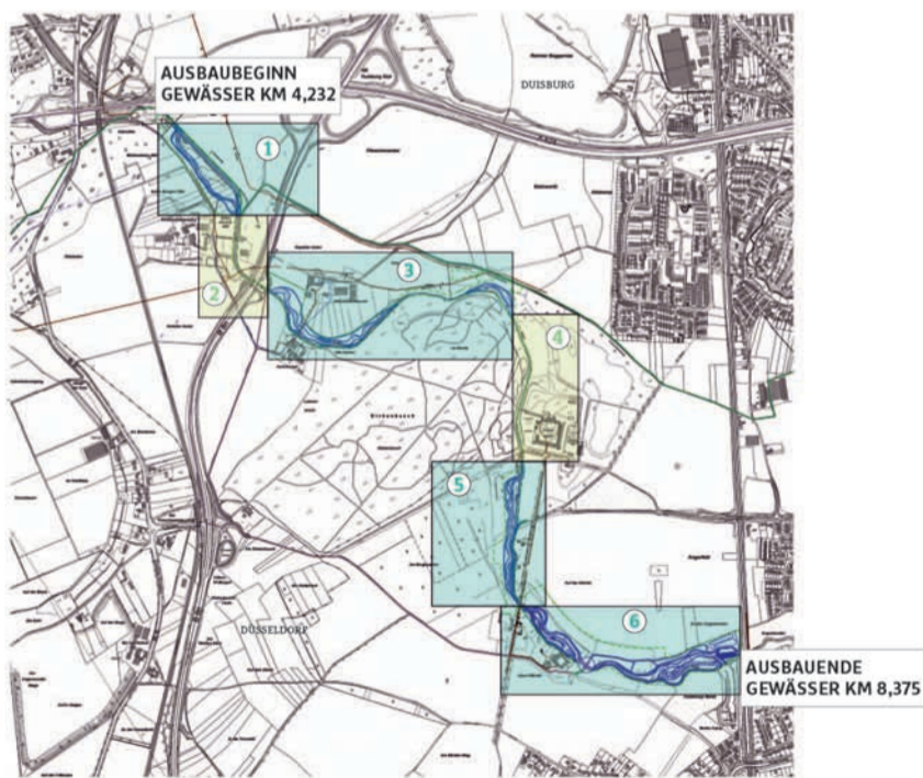
Übersichtsplan Sanierungsmaßnahmen in Angermund naturnaher Ausbau: Anger - Abschnitt I
